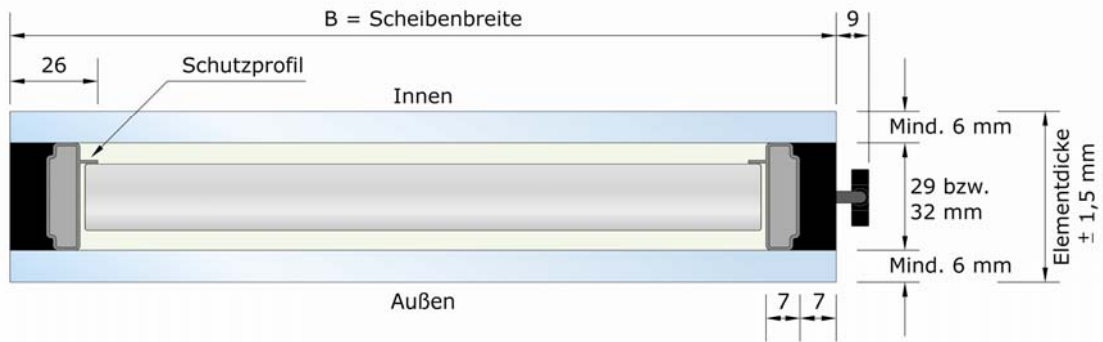
Schnitt ohne Kabel
