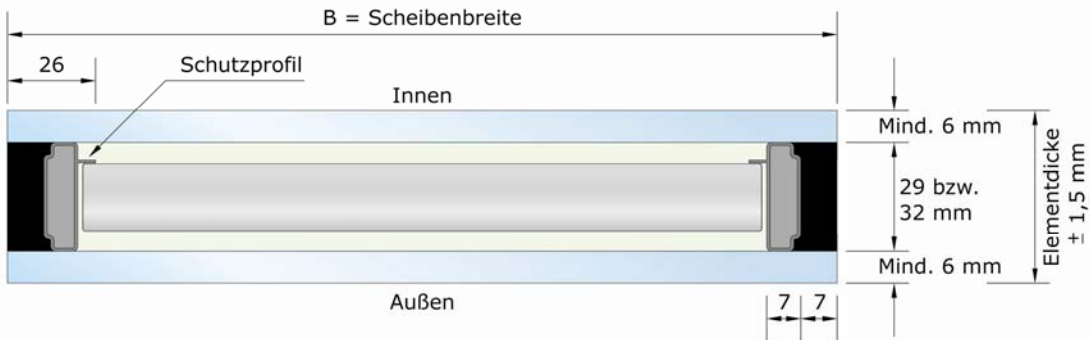
Schnitt ohne Kabel
