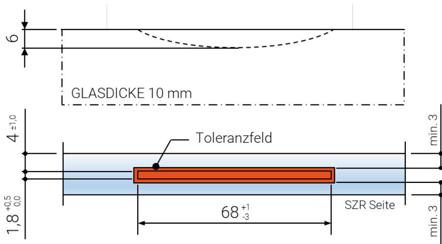
Abbildung 32: Toleranzen des Kantensegmenteinschliff bei 10 mm Glasdicke
