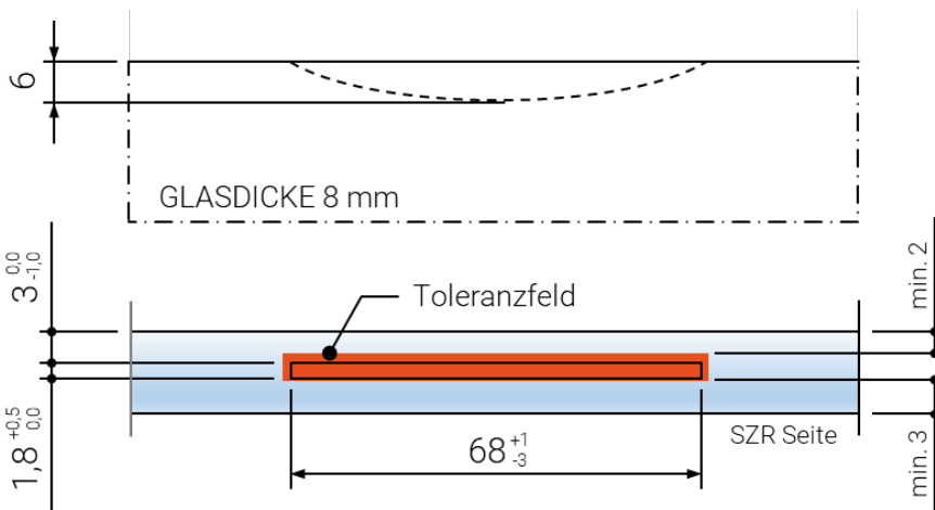
Abbildung 31: Toleranzen des Kantensegmenteinschliff bei 8 mm Glasdicke
