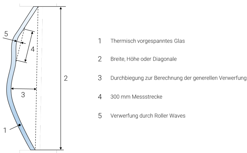
Abbildung 19: Darstellung der generellen Verwerfung und Verwerfung durch Roller Waves
