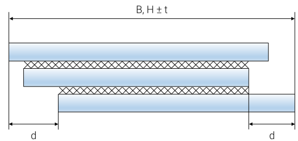
Abbildung 23: Versatz bei Verbundsicherheitsglas
