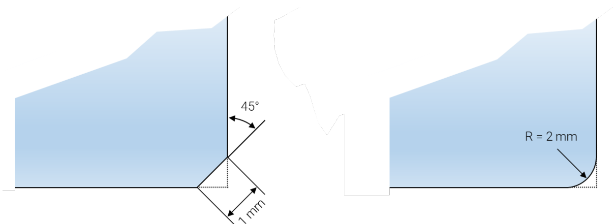
Abbildung 16: Eckstoß
