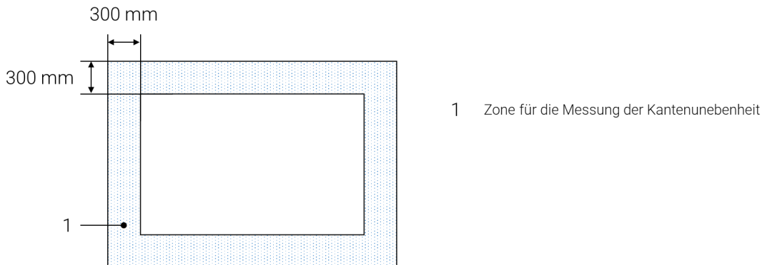
Abbildung 21: Zone für die Messung der Kantenunebenheit
