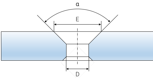
Abbildung 14: Senklochbohrung
