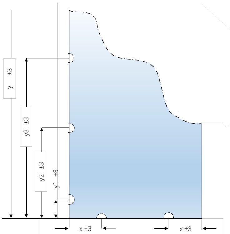
Abbildung 34: Lagetoleranz der Kantensegmenteinschliffe
