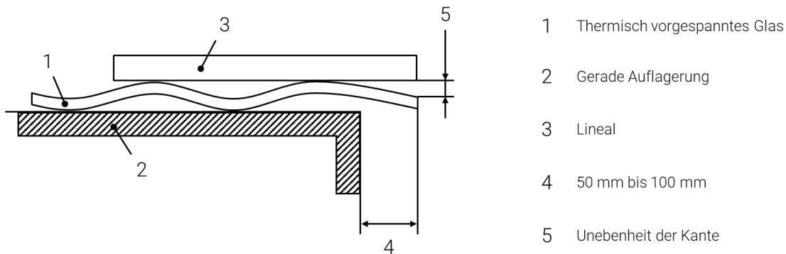
Abbildung 22: Messung der Unebenheit der Kanten
