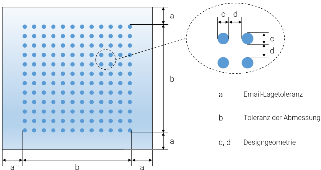
Abbildung 18: Lage- und Designtoleranzen bei bedruckten Gläsern
